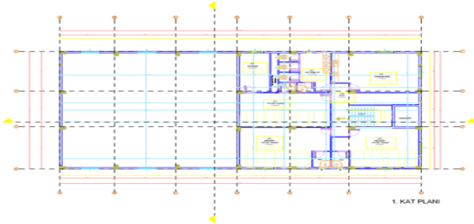
Şekil 51. Zafertepe İtfaiye Binası 1. Kat Planı
