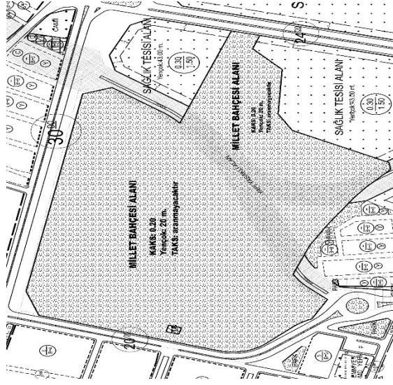
Harita 7. Millet Bahçesi İmar Planı
